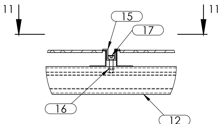
DETAL TYPOWY: ZAMOCOWANIE PANELA-KLEMA ŚRODKOWA SKALA 1 : 10
