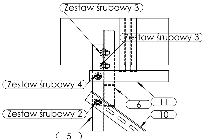
PRZEKRÓJ 6-6 SKALA 1 : 10
