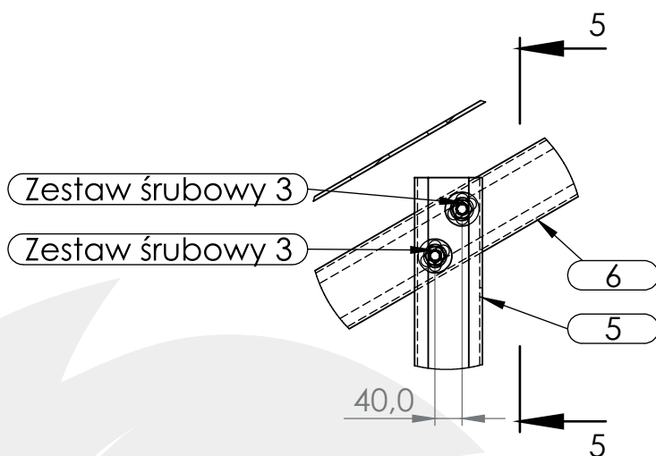
DETAL TYPOWY: POŁĄCZENIE PODPORA TYLNA - BELKA, POŁĄCZENIE PODPORA PRZEDNIA - BELKA SKALA 1 : 10
