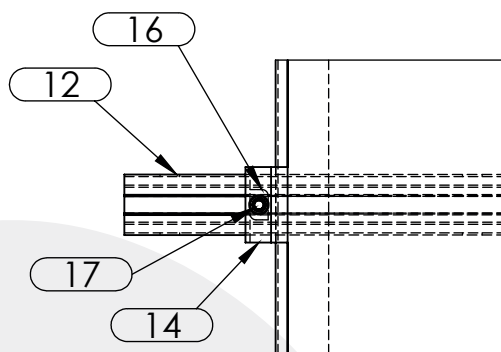
PRZEKRÓJ 12-12 SKALA 1 : 5
