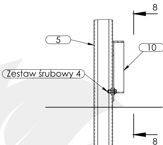
DETAL TYPOWY: POŁĄCZENIE PODPORA - STĘŻENIE (WĘZEL DOLNY) SKALA 1 : 10
