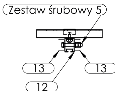
PRZEKRÓJ 9-9 SKALA 1 : 10
